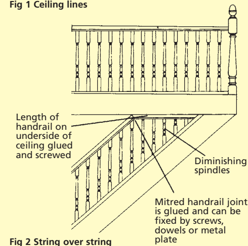
Fig 2 String over string
